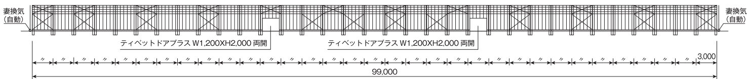
連棟側面図
