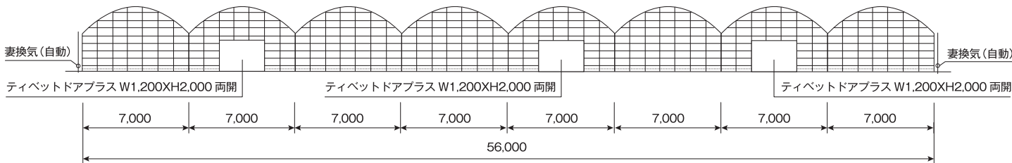
連棟正面図
